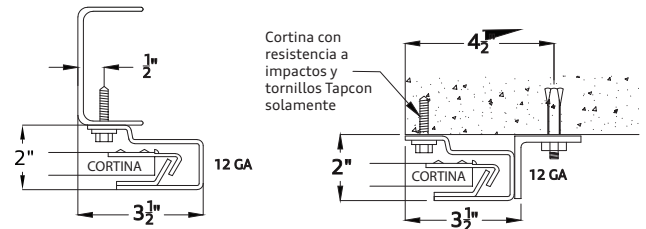
Montaje de detalles de las guías en acero
