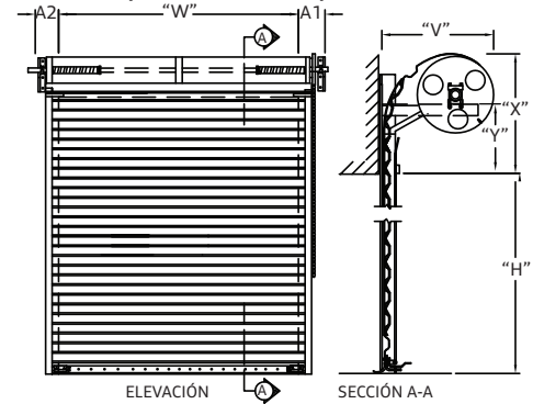
Montaje de detalles de las guías en acero
