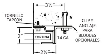
Montaje de guía estándar de 201 en mampostería
