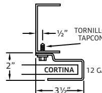
Montaje de guía estándar de 201 HD en acero
