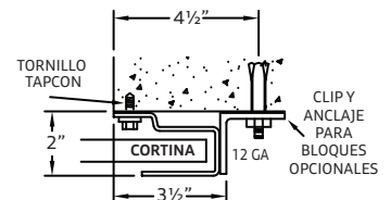
Montaje de guía estándar de 201 HD en mampostería
