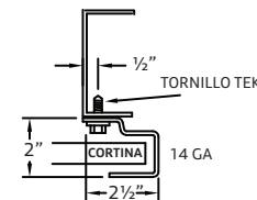
Montaje de guía estándar de 201 en acero
